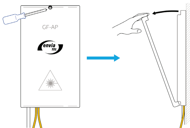
Bild 3: Deckel vom Gf-AP lösen
