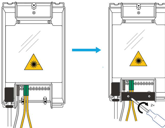
Bild 5: Gf-AP gesichert mit Zugentlastung
