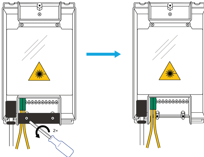
Bild 4: Gf-AP geöffnet mit Zugentlastung
