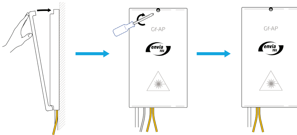
Bild 7: Gf-AP verschließen
