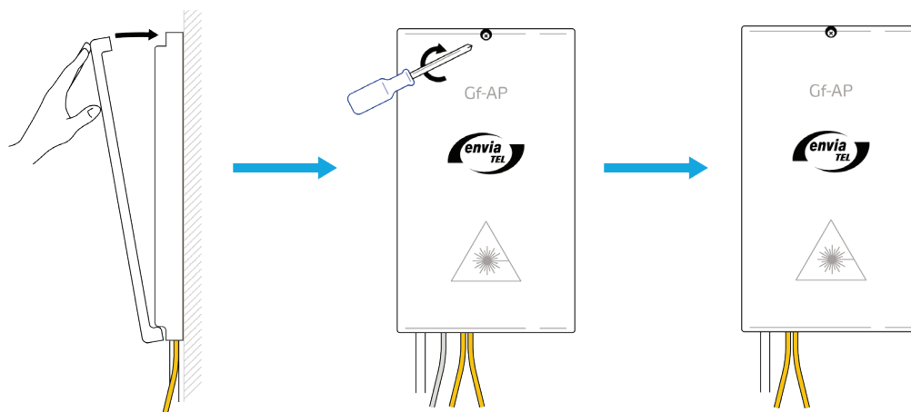
Bild 7: Gf-AP verschließen
